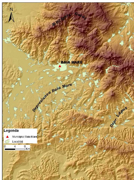
Fig. nr. 3 Harta formelor de relief în arealul Depresiunii Băii Mari
