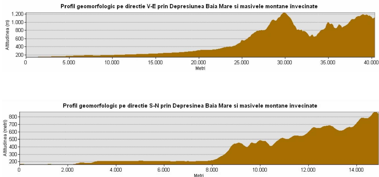
Fig. nr. 4 Profilele geomorfologice pe direcția V-E și S-N
