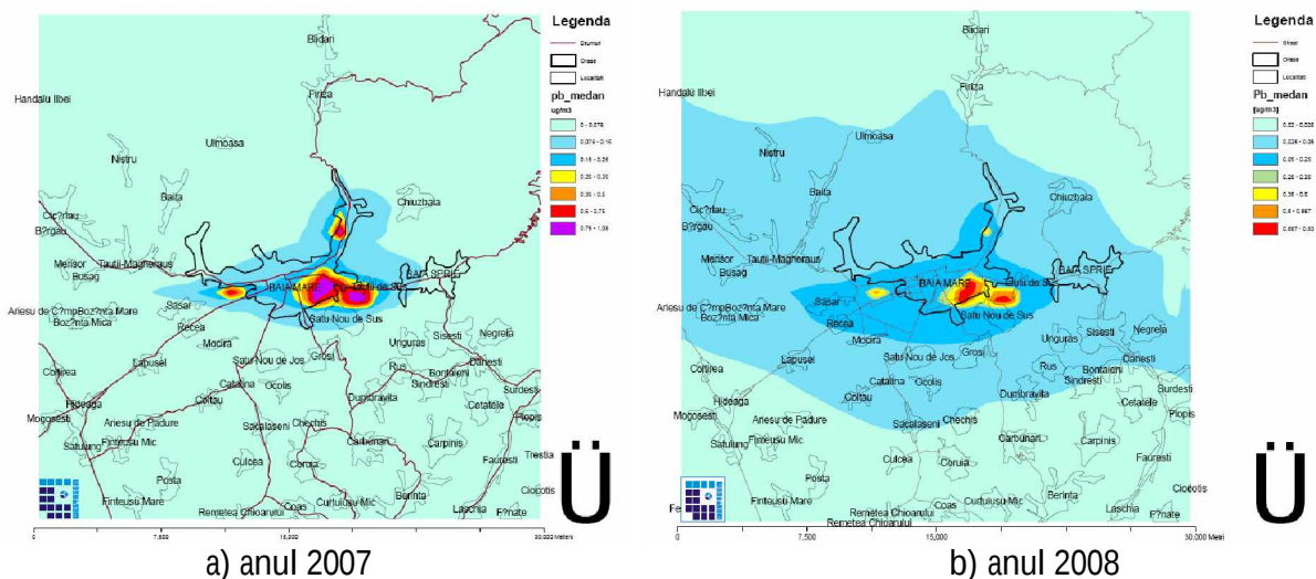
Fig. nr. 13 Distribuția spațială în aglomerarea Baia Mare a concentrației medii anuale de Pb din PM10 (din Studiul de evaluare a calității aerului în 2007 și 2008 realizat de WESTAGEM SRL București)
