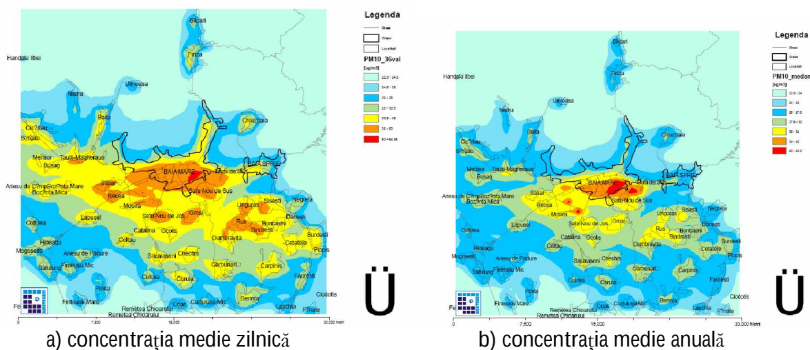
Fig. nr. 12 Distribuția spațială în aglomerarea Baia Mare a concentrației medii de PM10 în anul 2008 (din Studiu de evaluare a calității aerului în anul 2008 realizat de WESTAGEM SRL București)
